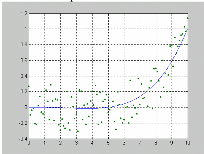
Gambar 1.3. Kurva Pendekatan
