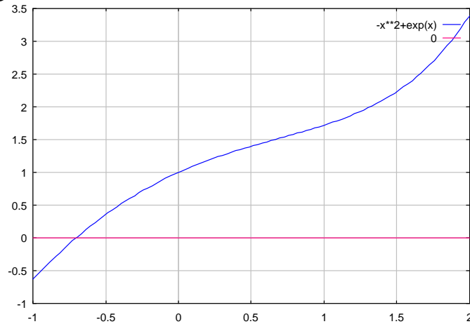
Gambar 1.2. Kurva y=x^2+exp(x)
